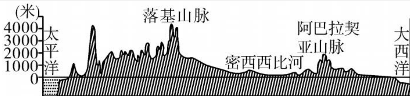
美国沿40°N地形剖面图
