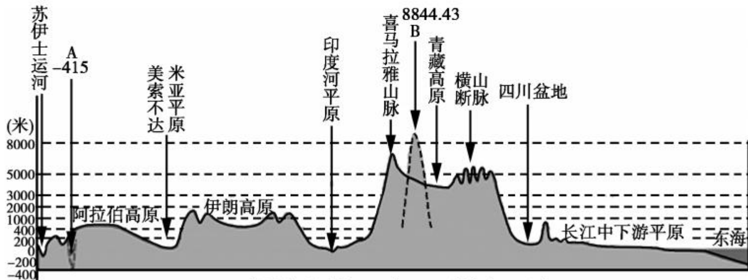
亚洲沿北纬30度地形剖面图
